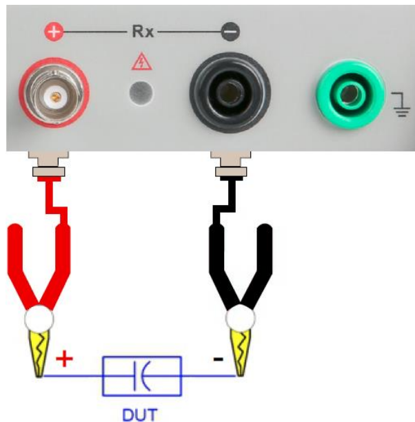
图 4-3 具有正负极的被测件的测量
