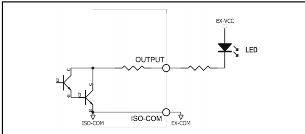
图 12-10 控制发光二极管或光电耦合器
