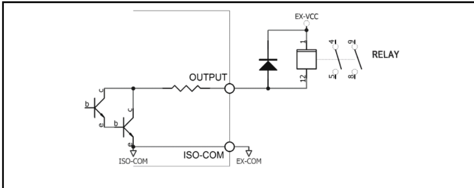
图 12-9 控制继电器
